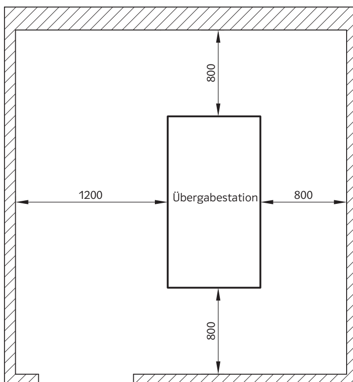
Freistehende Übergabestationen
